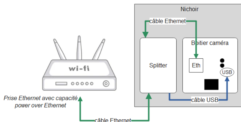
Figure 5 : Schéma de connexion du nichoir en power over Ethernet
