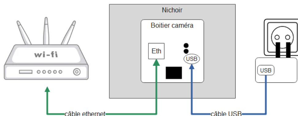
Figure 4 : Schéma de connexion du nichoir en Ethernet câblé + alimentation USB
