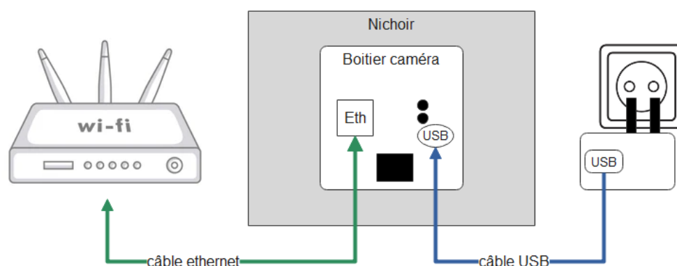
Figure 1 : Schéma de connexion du nichoir caméra au routeur pour la configuration
