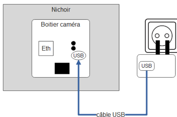
Figure 3 : Schéma de connexion du nichoir en WiFi
